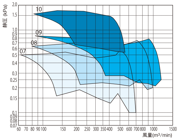
軸流型 A2D(7,8,9,10) 50Hz
