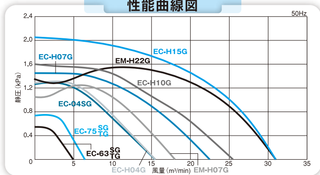
性能曲線図
