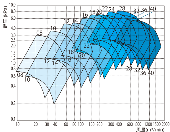
ターボ型 B3
