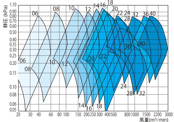
中圧プレート型 S2GP
