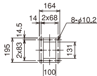
吐出相フランジ FB32x4.5
