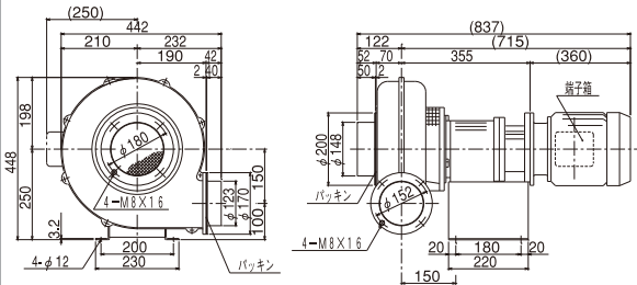
( ) 内寸法は電動機メーカーにより異なる場合があります。 EC-H10HT (0.75kW)
