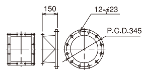
吐出連絡管 JIS 5K-250A オプション
