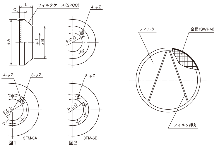
図1 図2 取付機種によって取付寸法が変わります。
