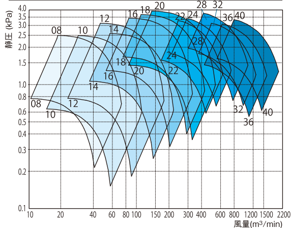
ターボ型 B2
