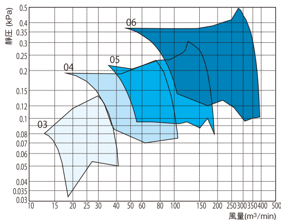
軸流型 A1D(7,8,9,10) 60Hz
