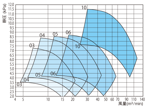
エアホイル型 S2KT
