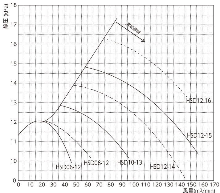
単段高压型性能曲線図 HSD(50/60Hz)
