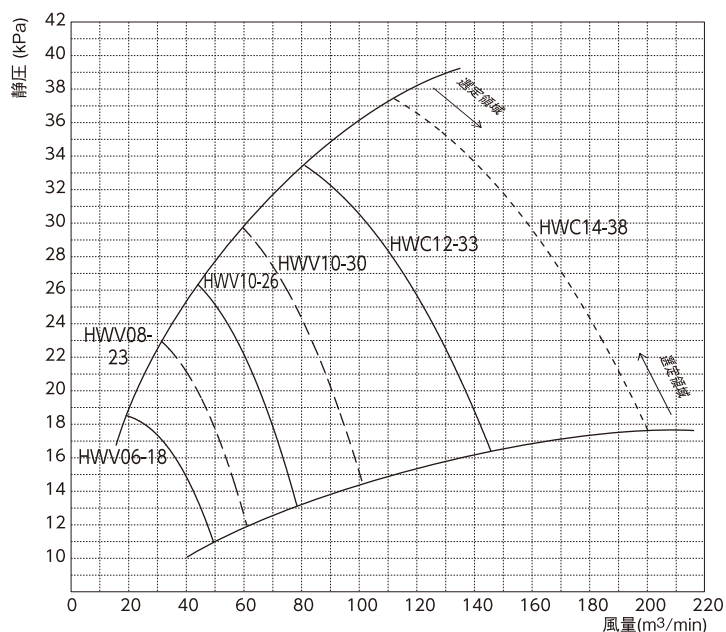
多段(段)高压型性能曲線図 HWV,HWC(50/60Hz)
