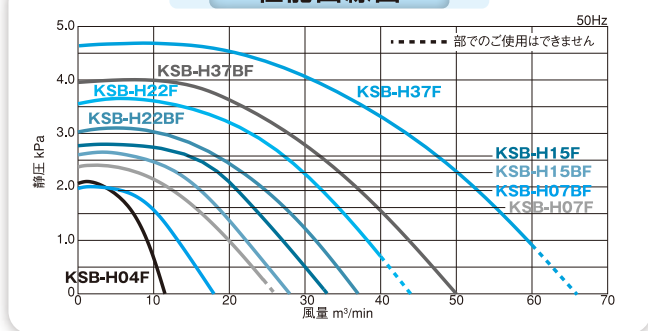
性能曲線図
