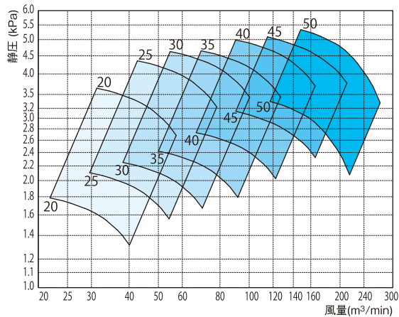
中圧プレート型 S2GP
