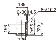
吐出相フランジ FB32x4.5
