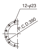
吸込口フランジ JIS 5K-300A
