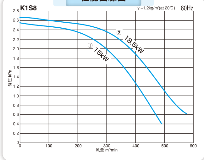
性能曲線図
