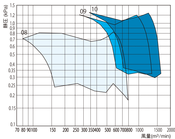
軸流型 A2D(7,8,9,10) 60Hz
