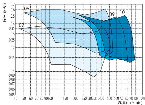
軸流型 A2D(3,4,5,6) 60Hz
