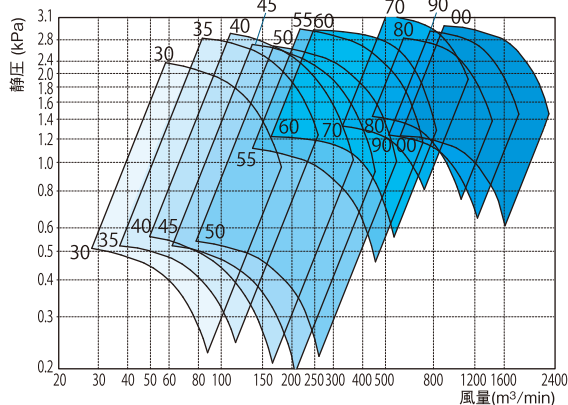
プレート型 P1
