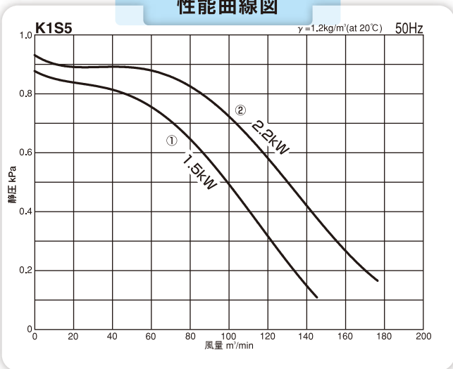
性能曲線図
