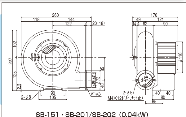
SB-151・SB-201/SB-202 (0.04kW)
