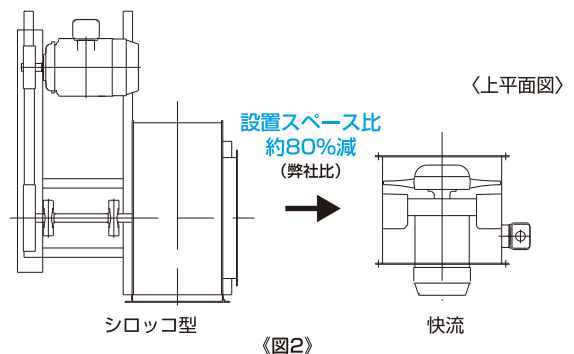
【同性能におけるシロッコ型との設置スペース比較】
