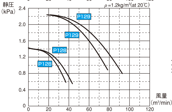
T1S形 (ターボ型) 左図T1S2~3 右図T1S4~5
