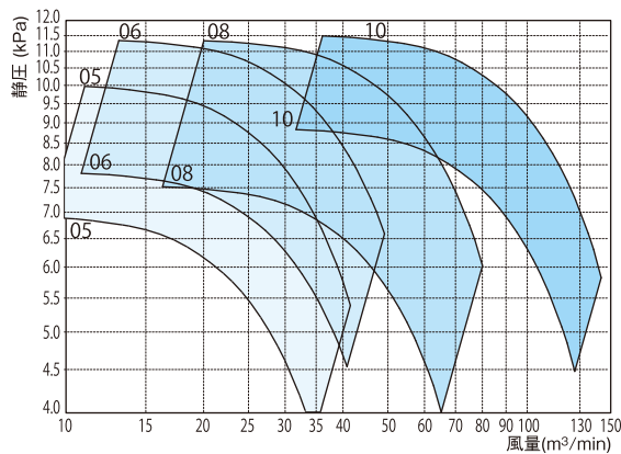
シロッコ型 M1
