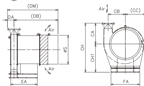
吐き出しフランジ JIS 5K
