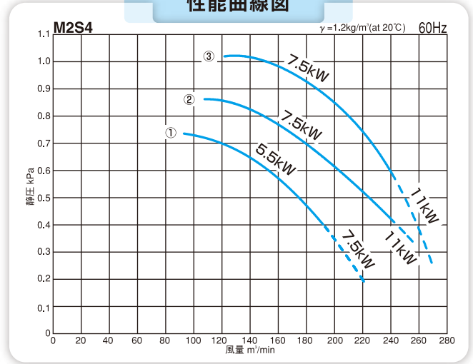
性能曲線図
