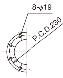
吸込口フランジ JIS 5K-150A
