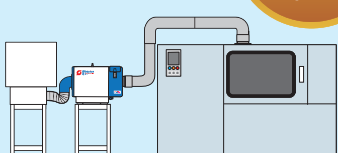
Instalación junto
