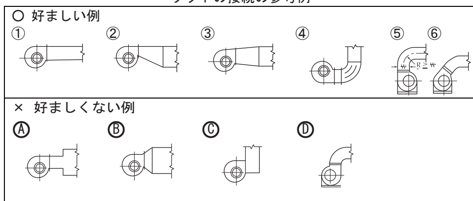
ダクトの接続の参考例
