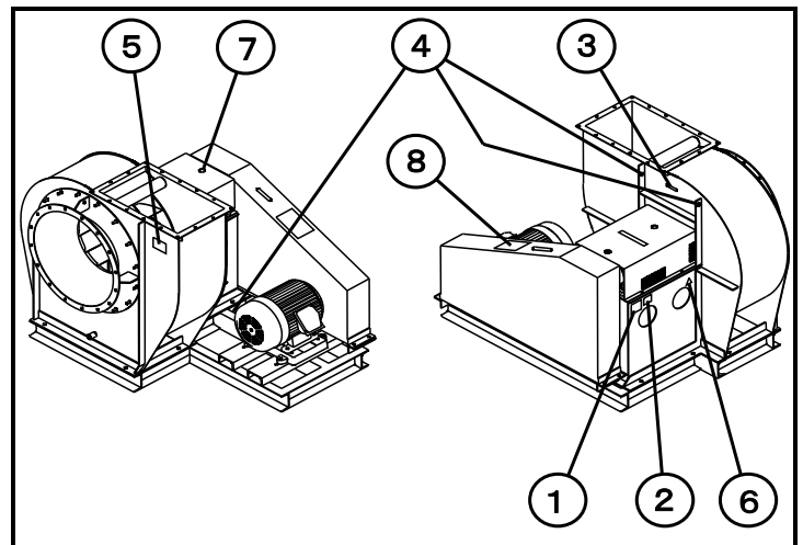
ベルト駆動外觀図
