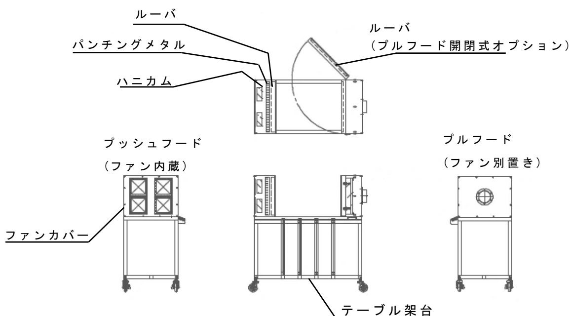
PPHT（水平流テーブル型）
